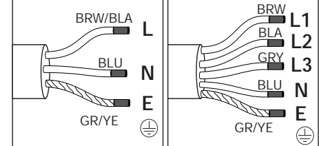
1 N AC 220-240 V
