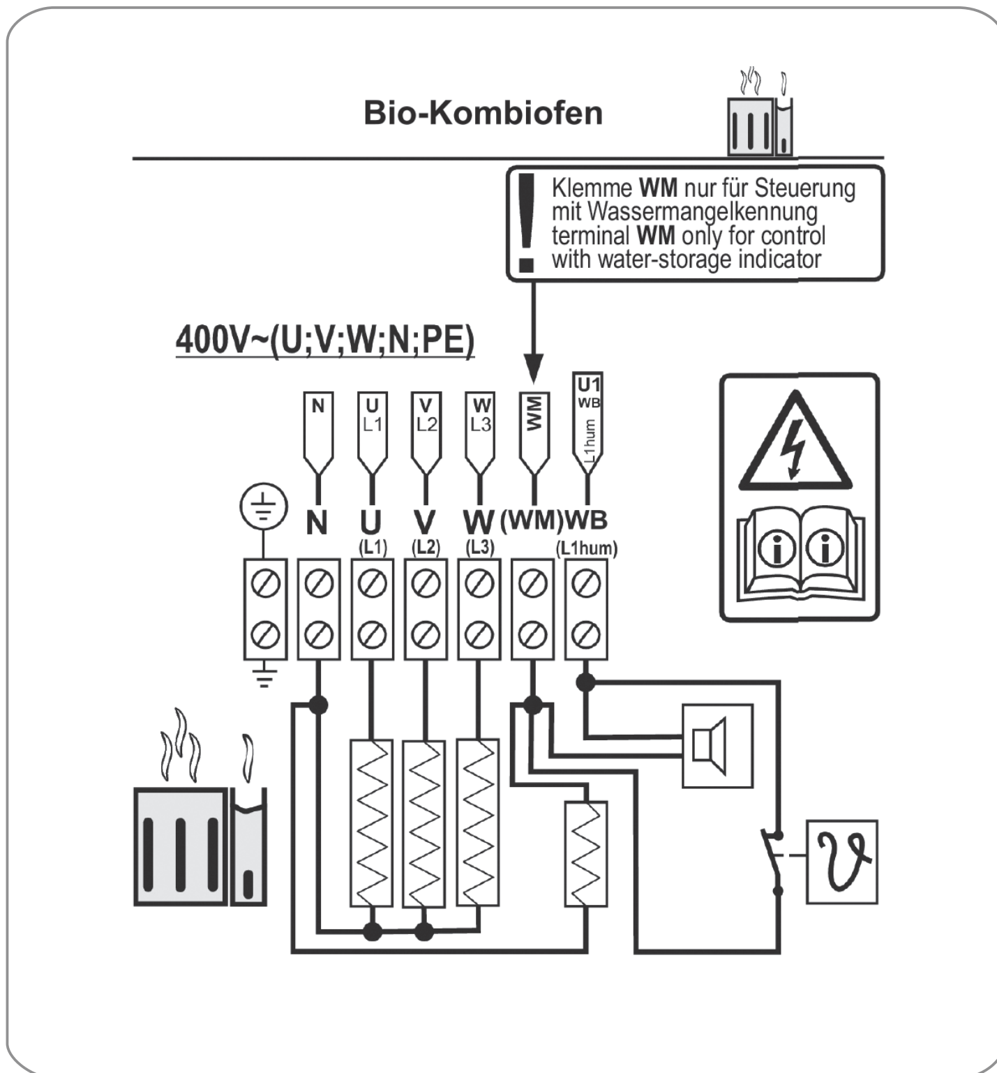
Anschlußplan Bio-Saunaofen
