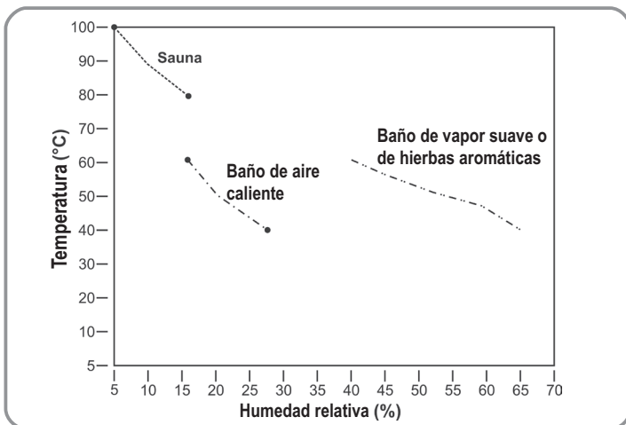
Formas de baño (diagrama de humedad/temperatura)
