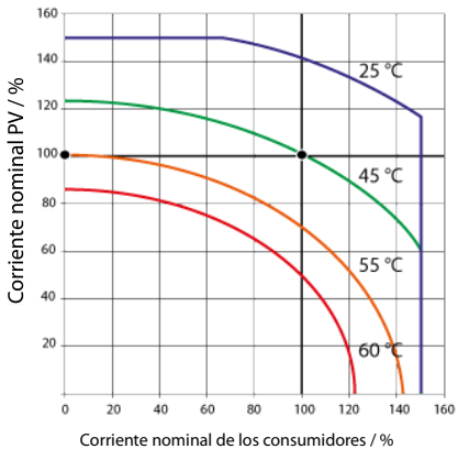
Zona de funcionamiento seguro de CXNup (SOA)
