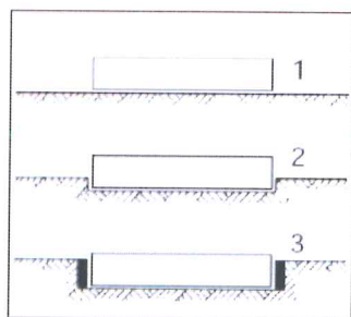
Rundformbecken
