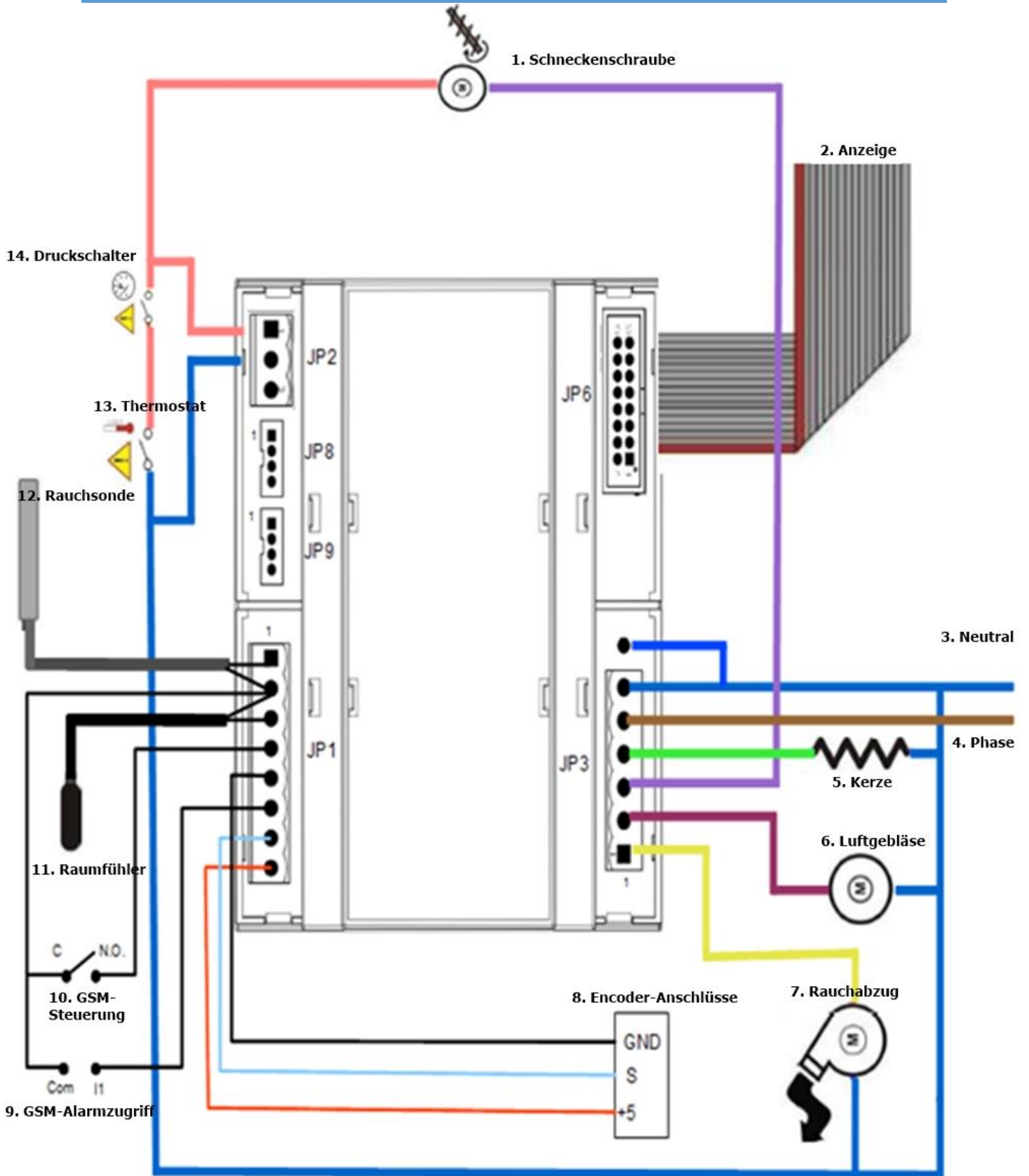
1: Schneckenschraube; 2: Anzeige; 3: neutral; 4: Phase; 5: Kerze; 6: Luftgebläse; 7: Rauchabzug; 8: Encoder-Anschlüsse; 9: GSM-Alarmzugriff; 10: GSM-Steuerung; 11: Raumfühler; 12: Rauchsonde; 13: Thermostat; 14: Druckschalter.
