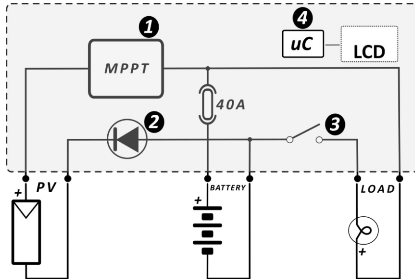
Abb.1 Prinzipschema
