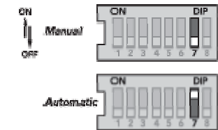
Abbildung 2.01 Schalter Nr. 7
