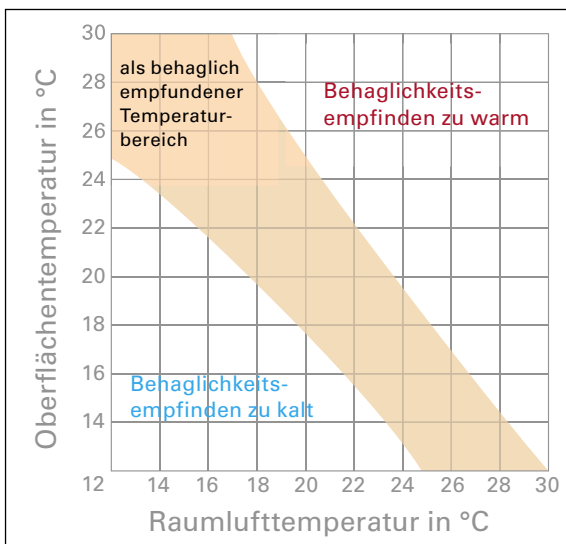
Temperaturabhängiges Behaglichkeitsempfinden
