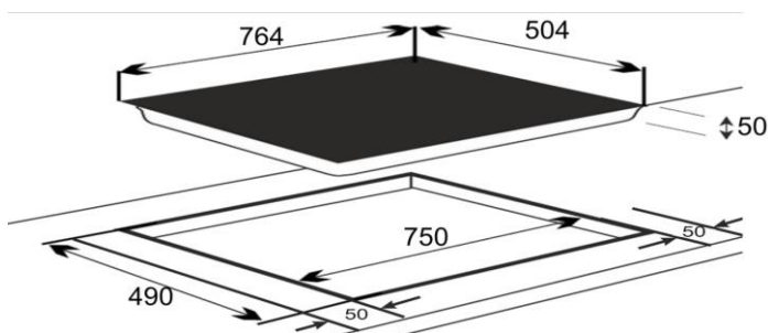
Einbauskizze
