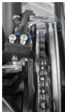
Aanslagschroef „High“ = voor grote kettingbladen
