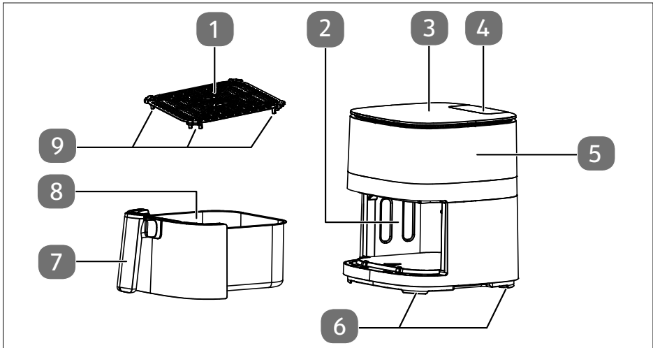
Abb. 1 - Vorderseite
