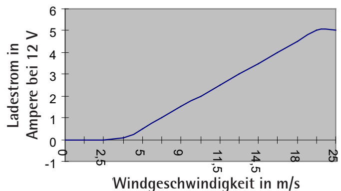
Leistungskurve „WG 504“
