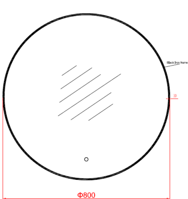
Vorderseite/Front
