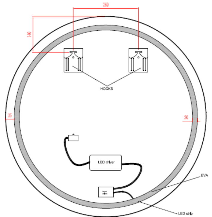
Rückseite/Backside
