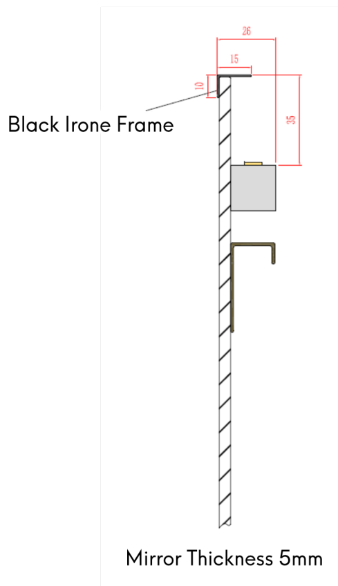
Seitenansicht/Sideview
