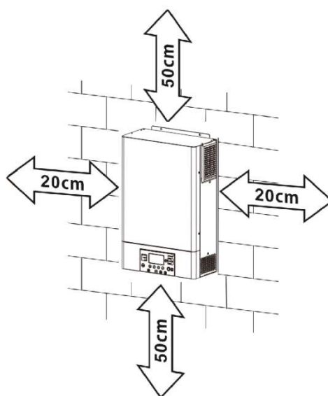
Abb. 5.1: Mindestabstand zu anderen Objekten
