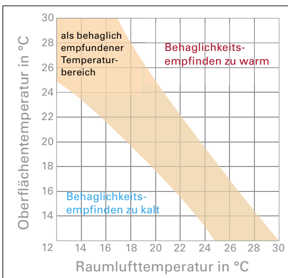
Temperaturabhängiges Behaglichkeitsempfinden
