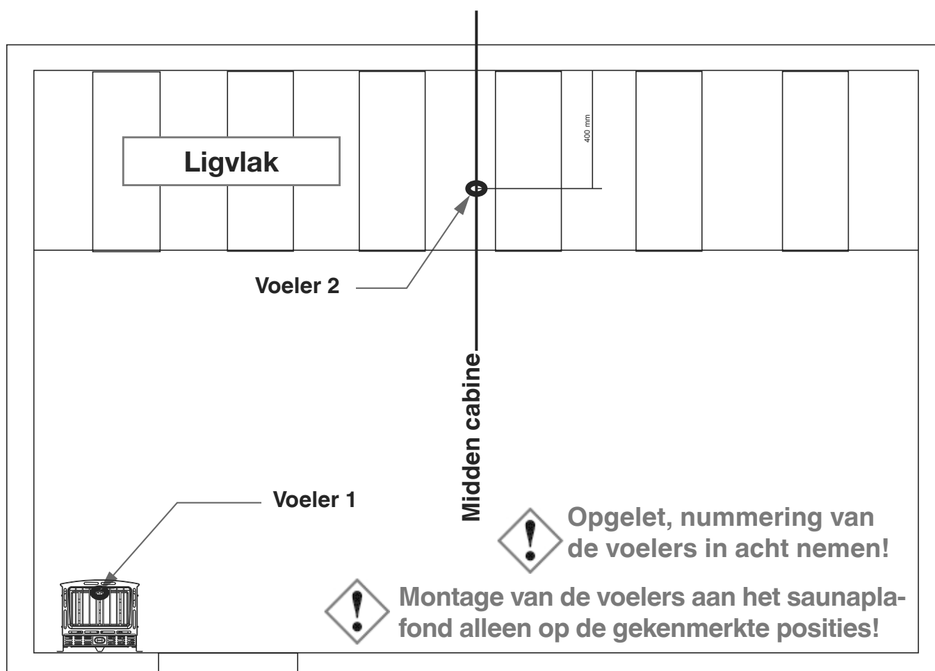
Bovenaanzicht – Saunacabines groter dan 8 m 3
