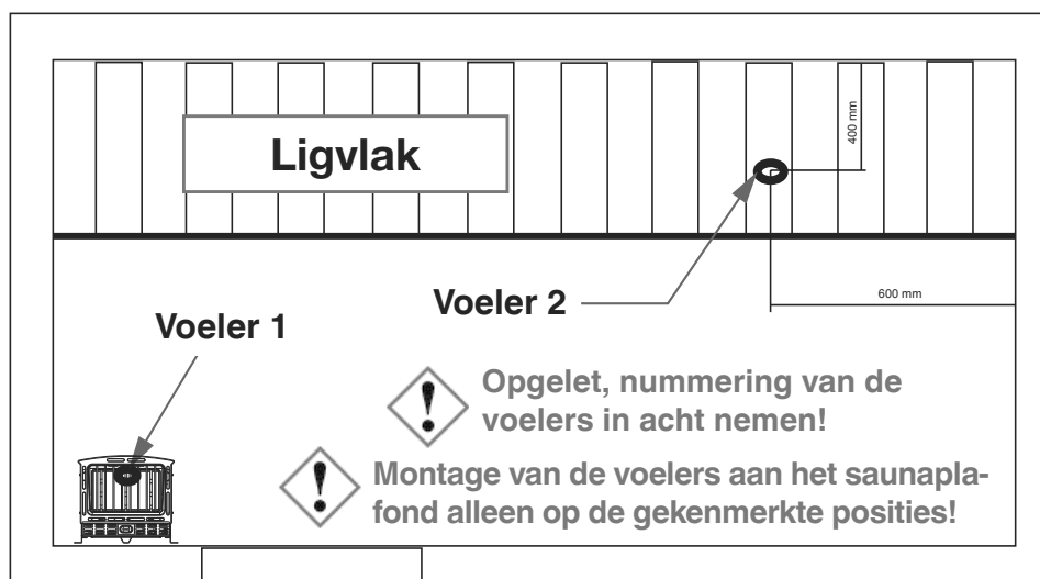
Bovenaanzicht – Saunacabines tot ca. 7,99 m 3
