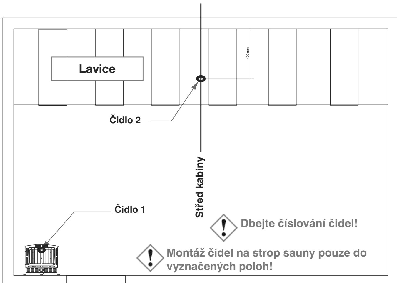
Půdorys – Saunové kabiny větší než 8 m 3
