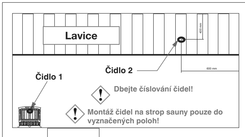
Půdorys – Saunové kabiny do cca 7,99 m 3
